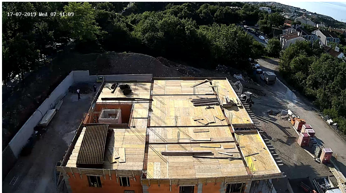
Slika 3: Snimka stanja radova pri početku snimanja (na dan 17.07.2019.)
