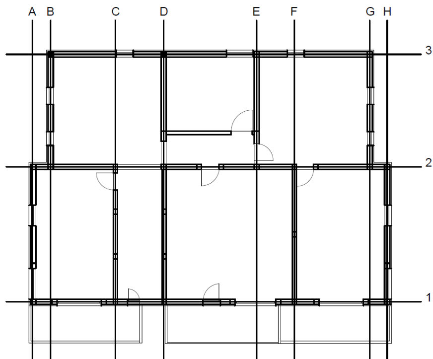
Slika 2: Tlocrt višestambene zgrade podijeljen na osi (1. kat) (Napomena: na shemi su prikazani samo zidani zidovi)
