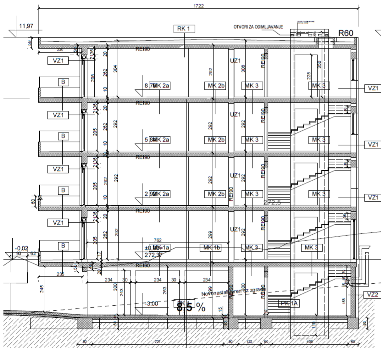
Slika 1: Višestambena zgrada, Kastav - Presjek A-A
