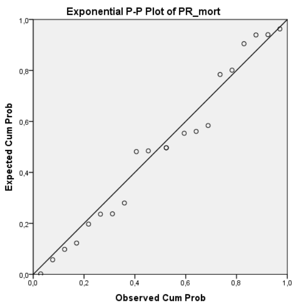
Slika 10 P-P plot dijagram za eksponencijalnu i gama distribuciju
