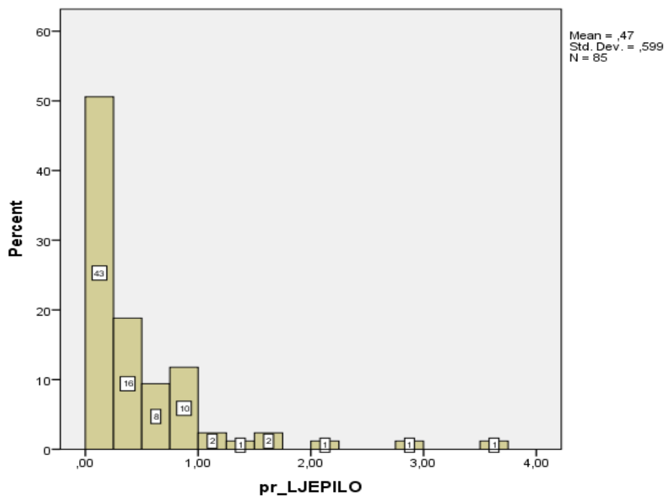
Slika 13 Dijagram frekvencija podataka rada pomoćnog radnika kod zidanja Porotherm Profi 30 opeke zidanje dry.fix ljepilom
