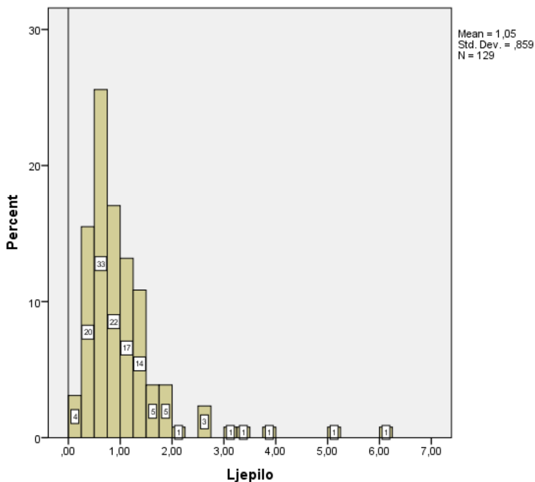
Slika 11 Dijagram frekvencija podataka za zidanje Porotherm Profi 30 opeke dry.FIX vezivnim sredstvom
