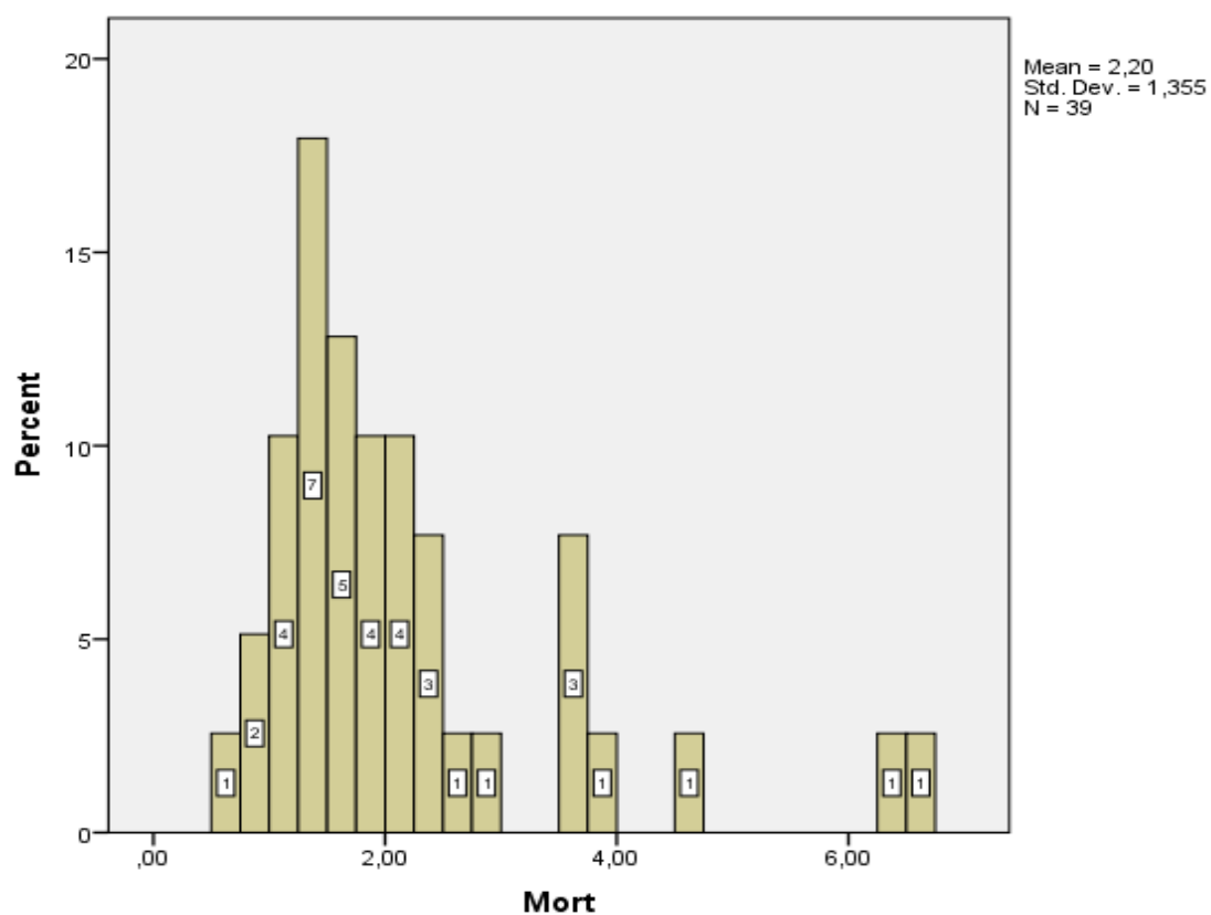
Slika 7 Dijagram frekvencija podataka za zidanje prvog reda Porotherm Profi 30 opeke
