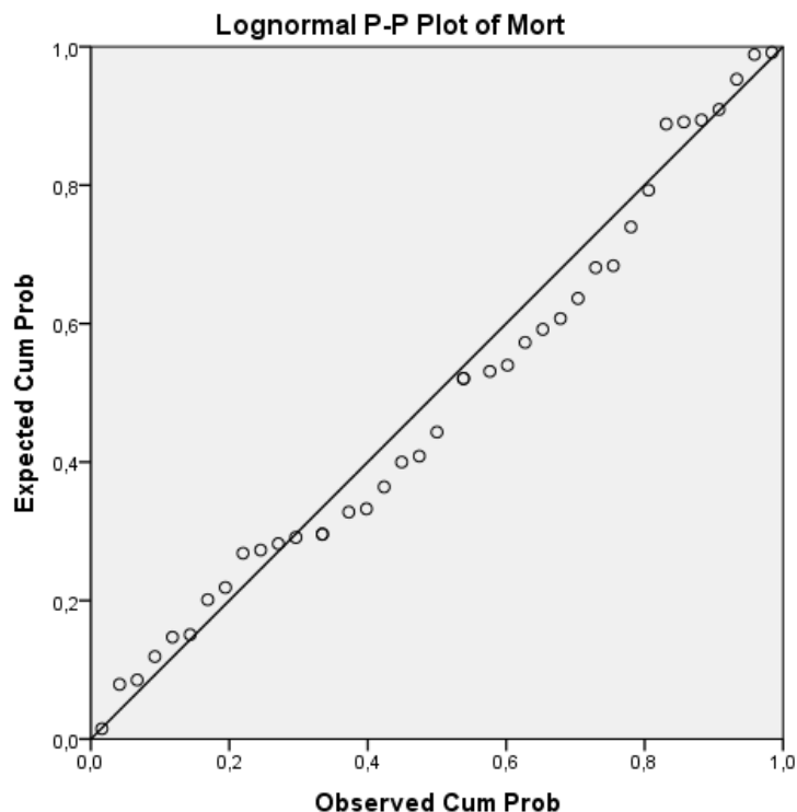
Slika 8 P-P plot dijagram za lognormalnu distribuciju
