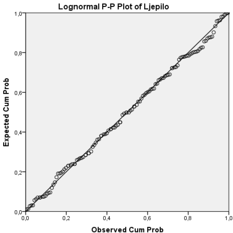
Slika 12 P-P plot dijagram za lognormalnu distribuciju
