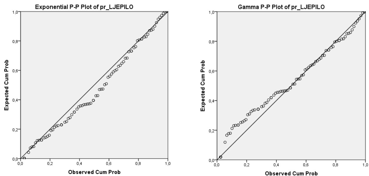
Slika 14 P-P plot dijagram za eksponencijalnu i gama distribuciju
