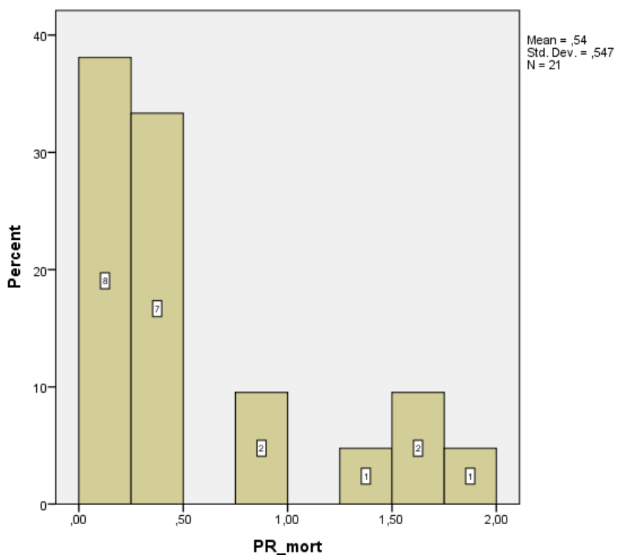
Slika 9 Dijagram frekvencija podataka rad pomoćnog radnika kod zidanja prvog reda Porotherm Profi 30 opeke
