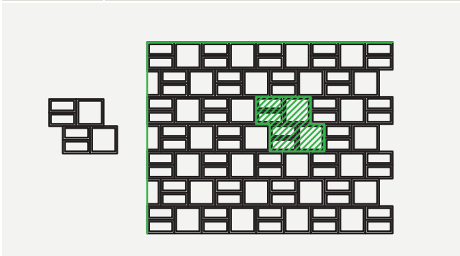
HEMA 3 Potrebno na m 2 : 20 x 20 x 10 cm - 12,5 kom. 10 x 20 x 10 cm - 25 kom.
