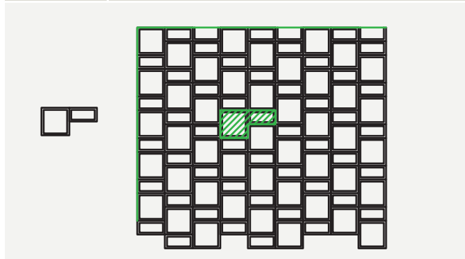
HEMA 4 Potrebno na m 2 : 20 x 20 x 10 cm - 16,66 kom. 10 x 20 x 10 cm - 16,66 kom.
