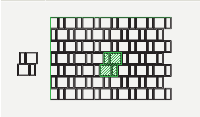
HEMA 5 Potrebno na m 2 : 20 x 20 x 10 cm - 8,33 kom. 10 x 20 x 10 cm - 8,33 kom.
